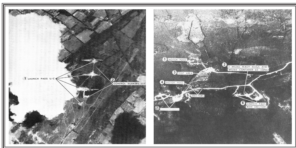
Fig. 19 Cuadro izquierdo: foto del emplazamiento en preparación para cohetes R-14; cuadro derecho: emplazamiento de uno de los grupos de combate del regimiento en la región central de la Isla.
